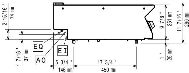
Zij aanzicht
